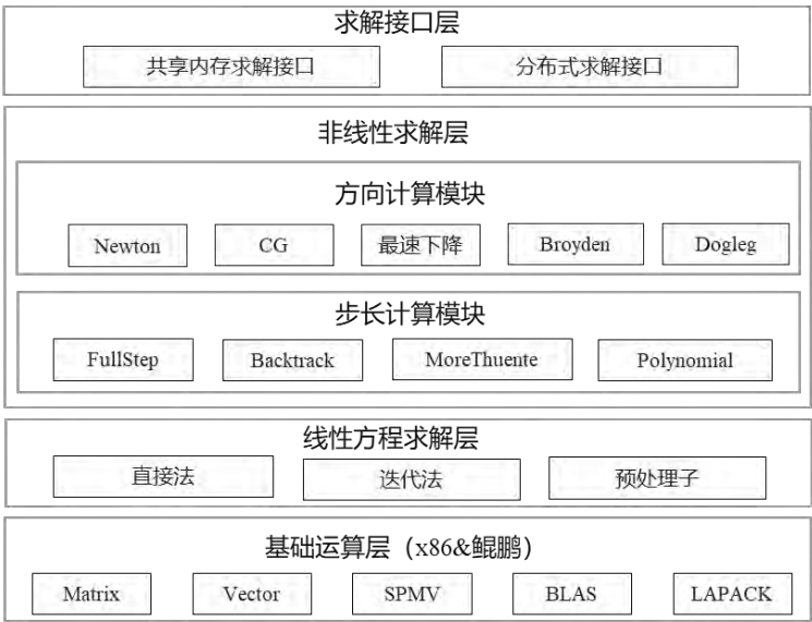
图2.37 非线性方程组求解器软件架构
