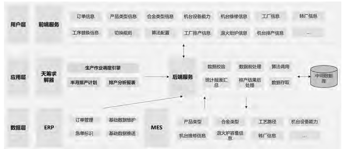
图4.19 应用架构及调用关系示意图
