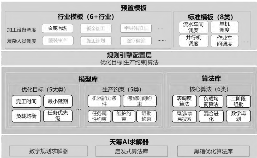
图3.6 生产调度求解器技术架构图
