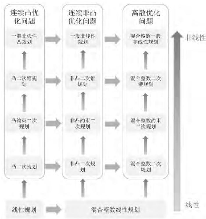
图2.3 数学规划问题分类
