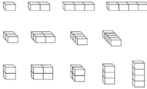
图3.17 三维装箱中“块”的概念示例说明
