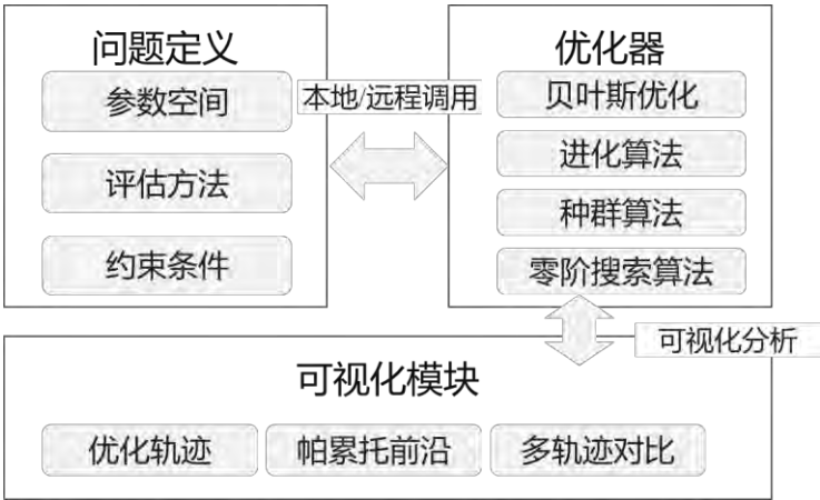
图2.18 黑箱优化求解器软件架构
